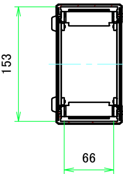
A-A ( 1 : 5 )
