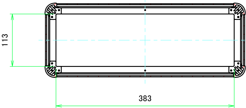
C-C ( 1 : 5 )
